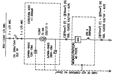
DIAGRAMA LÂMPADA SEM ESCALA
